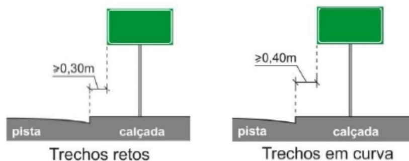
FIGURA 14 – Afastamento Lateral da Placa.
