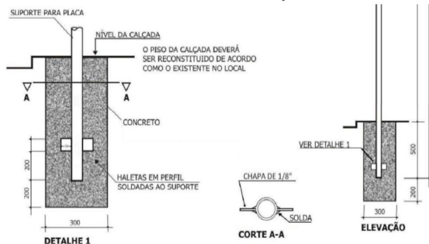
FIGURA 12 – Detalhe da Fundação.
