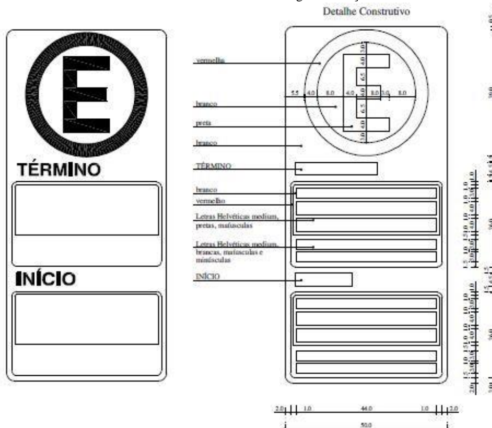
FIGURA 5 – Modelo de Placa de Regulamentação.
