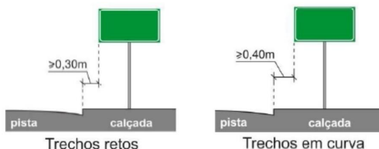
FIGURA 11 – Afastamento Lateral das Placas.
